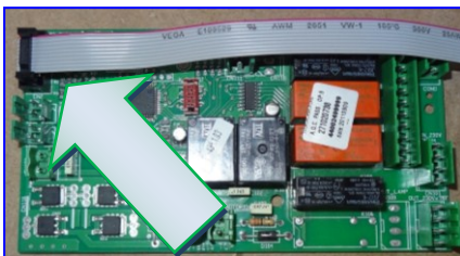
Collegamento pulsantiera SDD2
